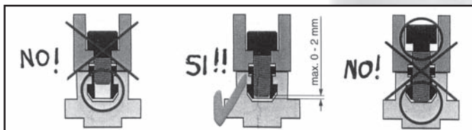
ESEMPIO CORRETTO DI MONTAGGIO DELLE VITI FRA MORSETTO E TASSELLO
